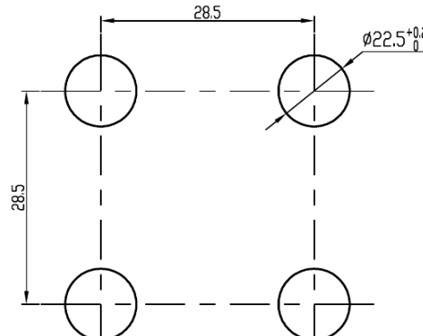
Montaj Delikleri
