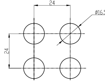
Montaj Delikleri
