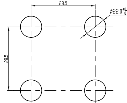
Montaj Delikleri
