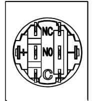
Klemens Düzeni
